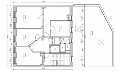
1 étage 1:100
