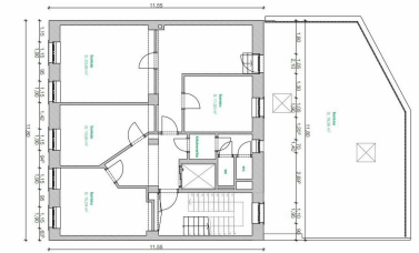
1 étage 1:100
